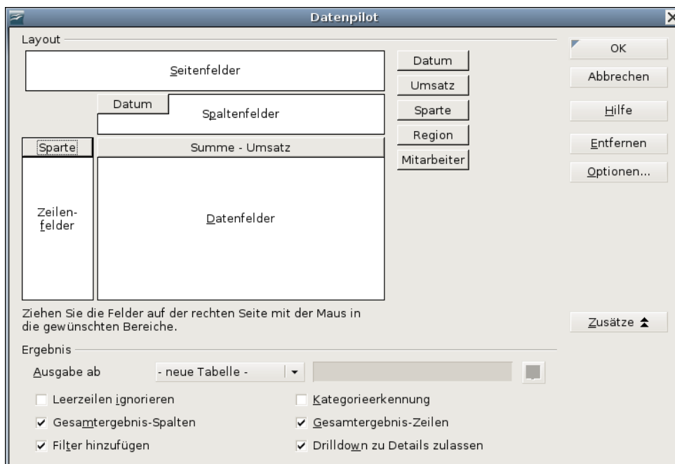
Abbildung 3: Dialog Datenpilot
