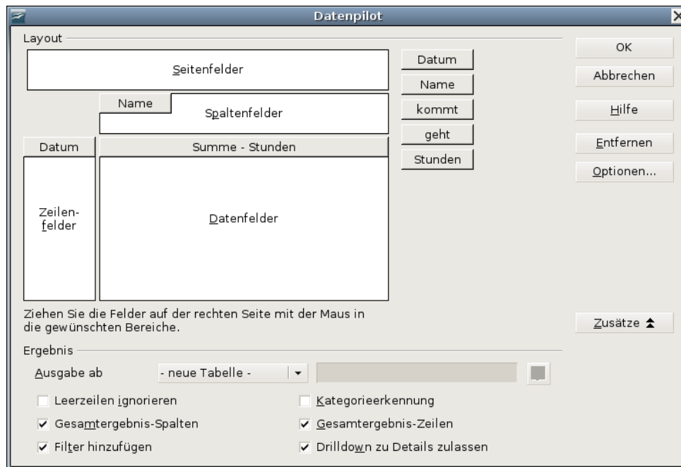
Abbildung 13: Dialog Datenpilot
