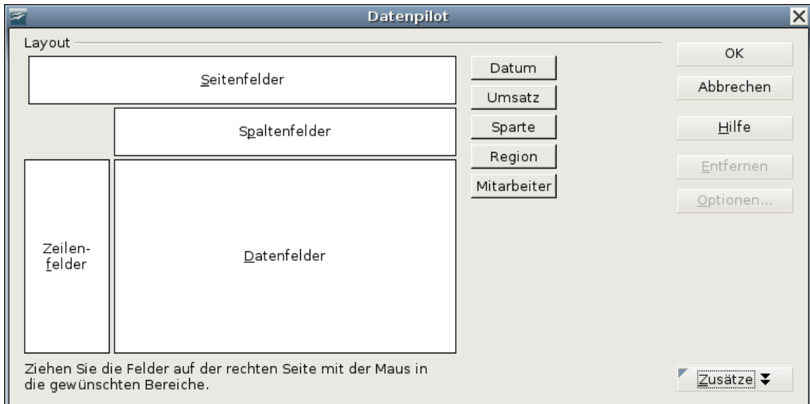
Abbildung 33: Dialog Datenpilot
