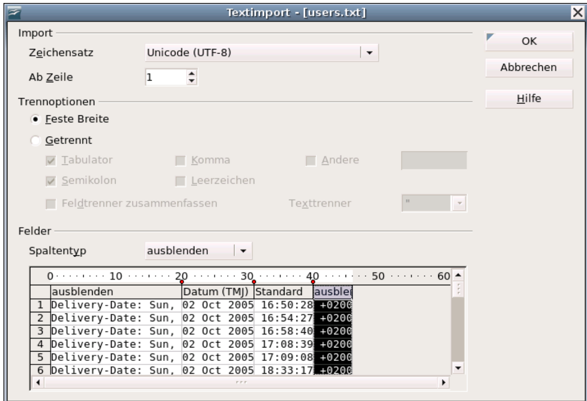
Abbildung 23: Import-Einstellungen
